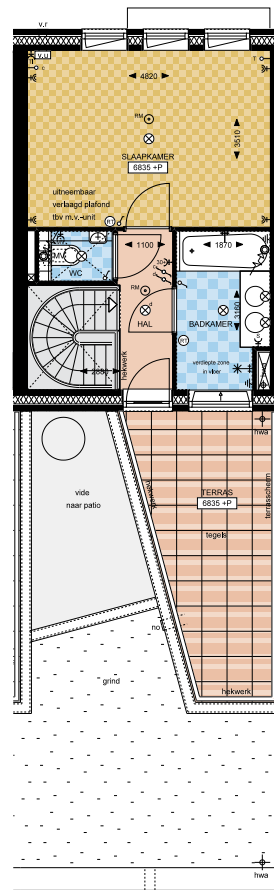
Tweede verdieping
