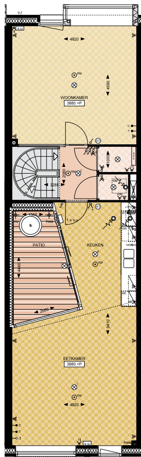
Eerste verdieping
