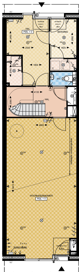
Begane grond
