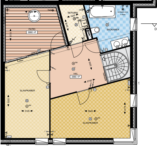
Eerste verdieping
