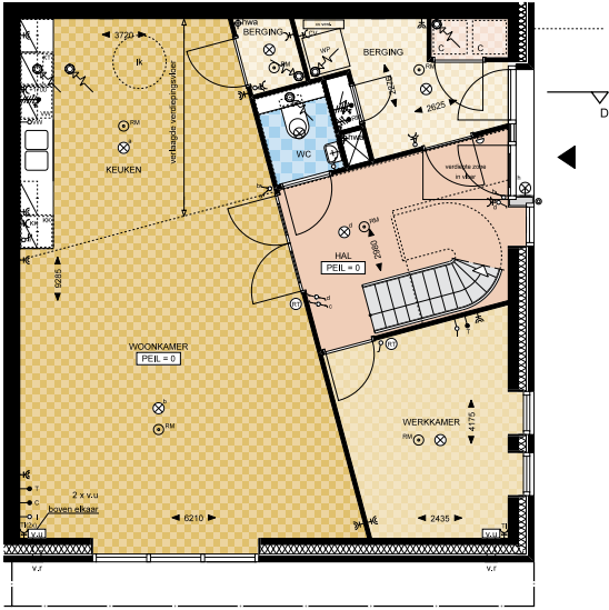
Begane grond
